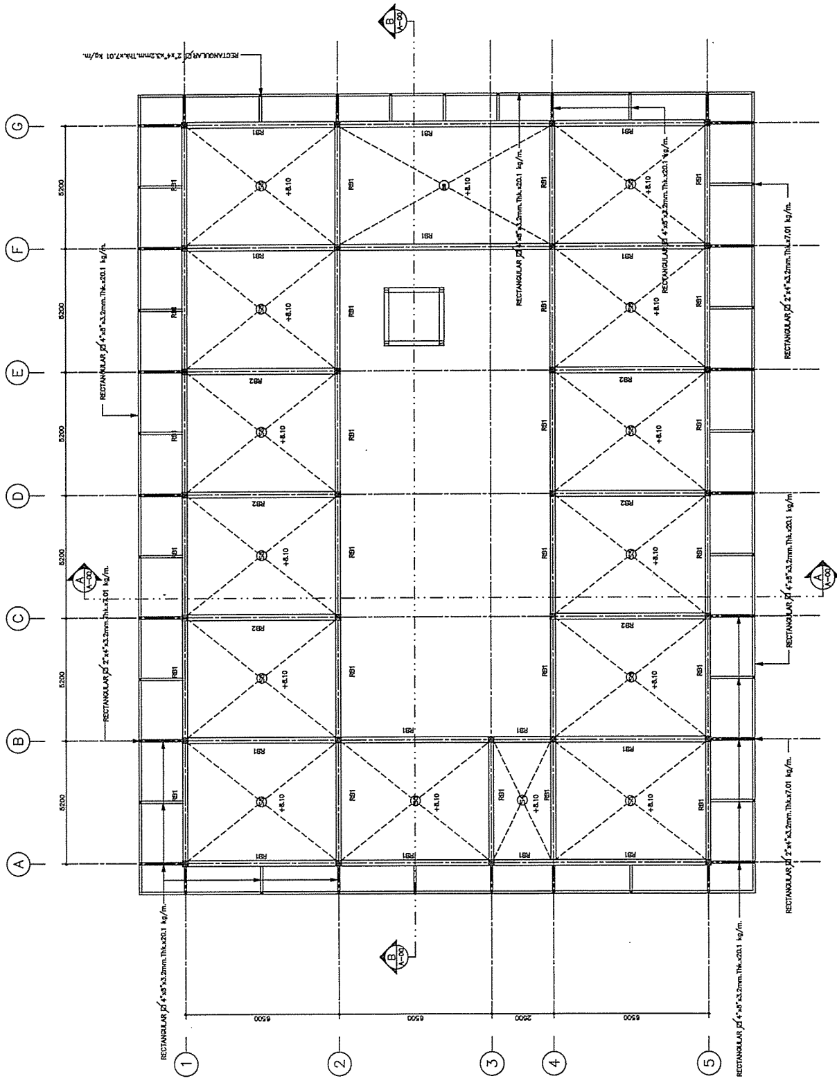
แปลน ตาแหน่ง ขอบอาคาร ชั้นหลังคา ระดับ +8.10 หน้าตัด
