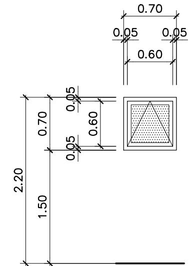
รูปด้าน W5 scale 1: 50
