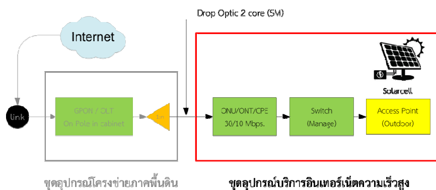
ภาพที่ 8 การเชื่อมต่อชุดอุปกรณ์ WiFi ชนิดโครงข่ายภาคพื้นดินแบบ ไม่มีไฟฟ้า
