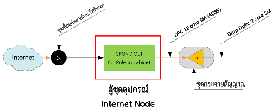
ภาพที่ 3 การติดตั้งและเชื่อมสัญญาณผ่านโครงข่ายภาคพื้นดิน ในจุดติดตั้งที่มีไฟฟ้า
