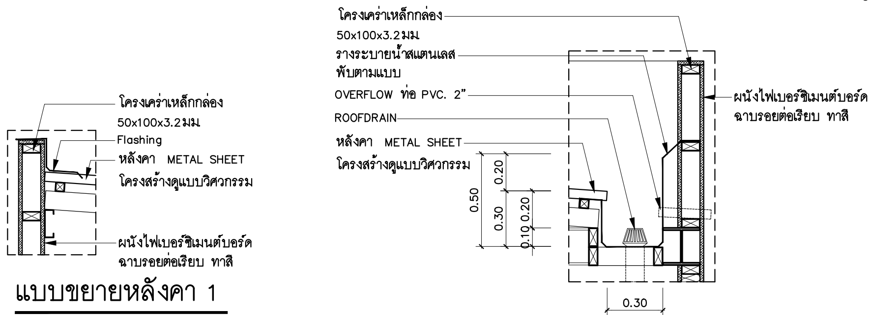
แบบขยายวางระบายนํ้าหลังคา scale 1:20
