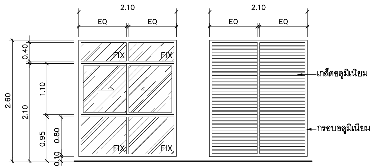
รูปด้าน W2 scale 1: 50
