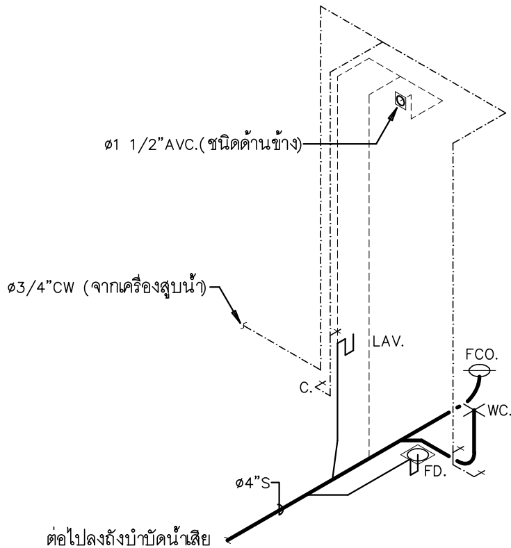
ไอโซเมตริกระบบสุขาภิบาลห้องน้ำ scale
