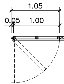
แปลน D5
