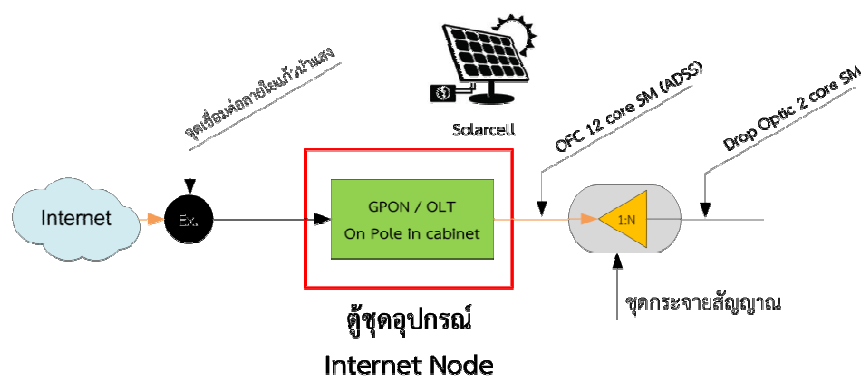
ภาพที่ 4 การติดตั้งและเชื่อมต่อสัญญาณผ่านโครงข่ายภาคพื้นดิน ในจุดติดตั้งที่ไม่มีไฟฟ้า
