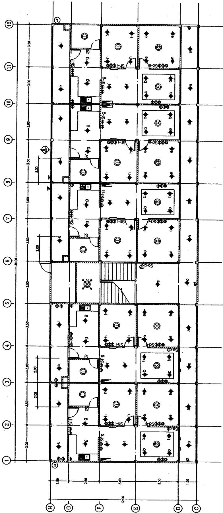
แปลนไฟฟ้าชั้นสอง ขนาดหน้า 1:125
