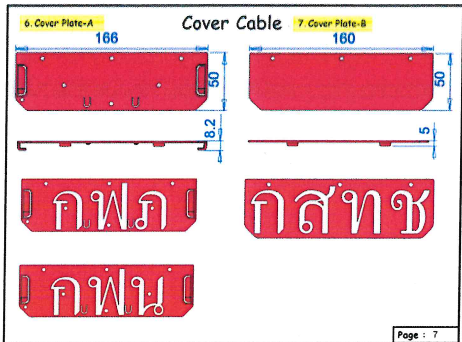
รูปที่ ๖ แสดงขนาดของป้ายทั้ง ๒ อัน
