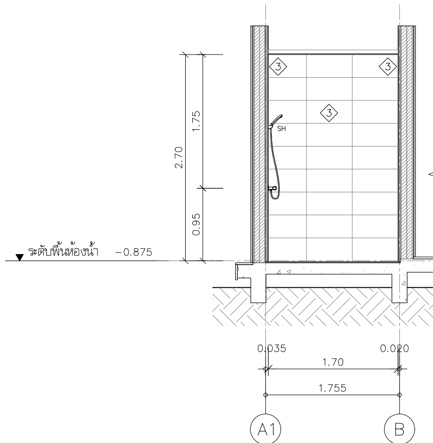
แบบขยายห้องน้ำ รูปตัด มาตราส่วน 1:50
