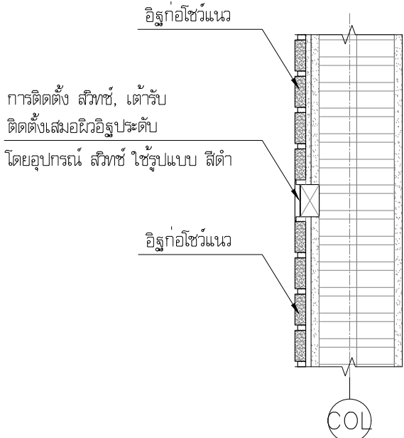
แบบขยาย การติดตั้งสวิตช์, เต้ารับ งานระบบไฟฟ้า มาตราส่วน 1:10
