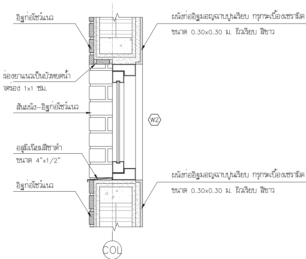
แบบขยาย การจบรอยต่อช่องเปิดหน้าต่าง มาตราส่วน 1:10
