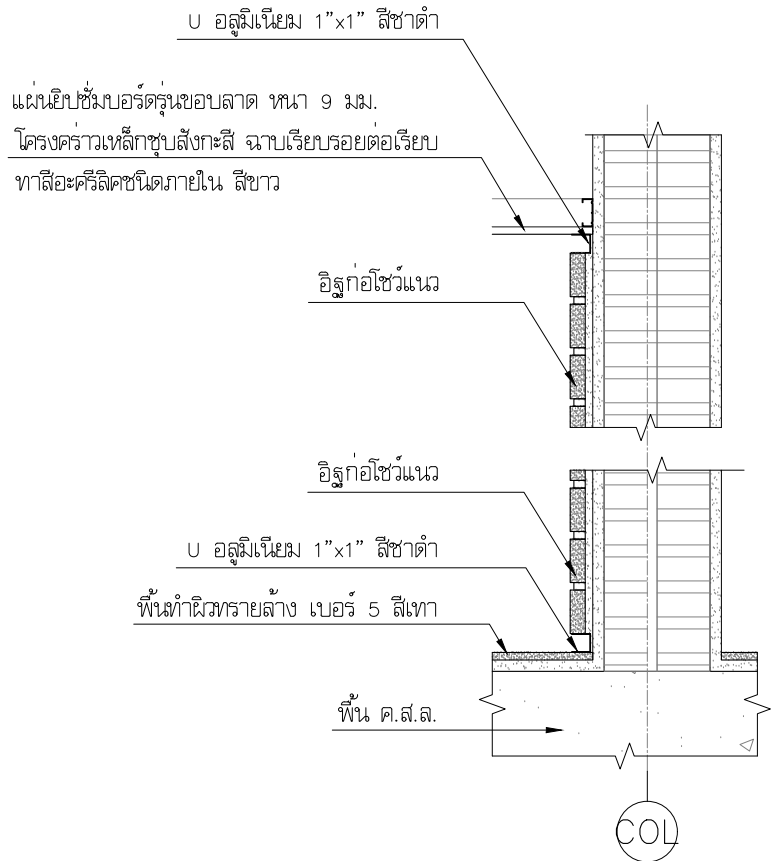
แบบขยาย การจบรอยต่อผนังกั้น มาตราส่วน 1:10
