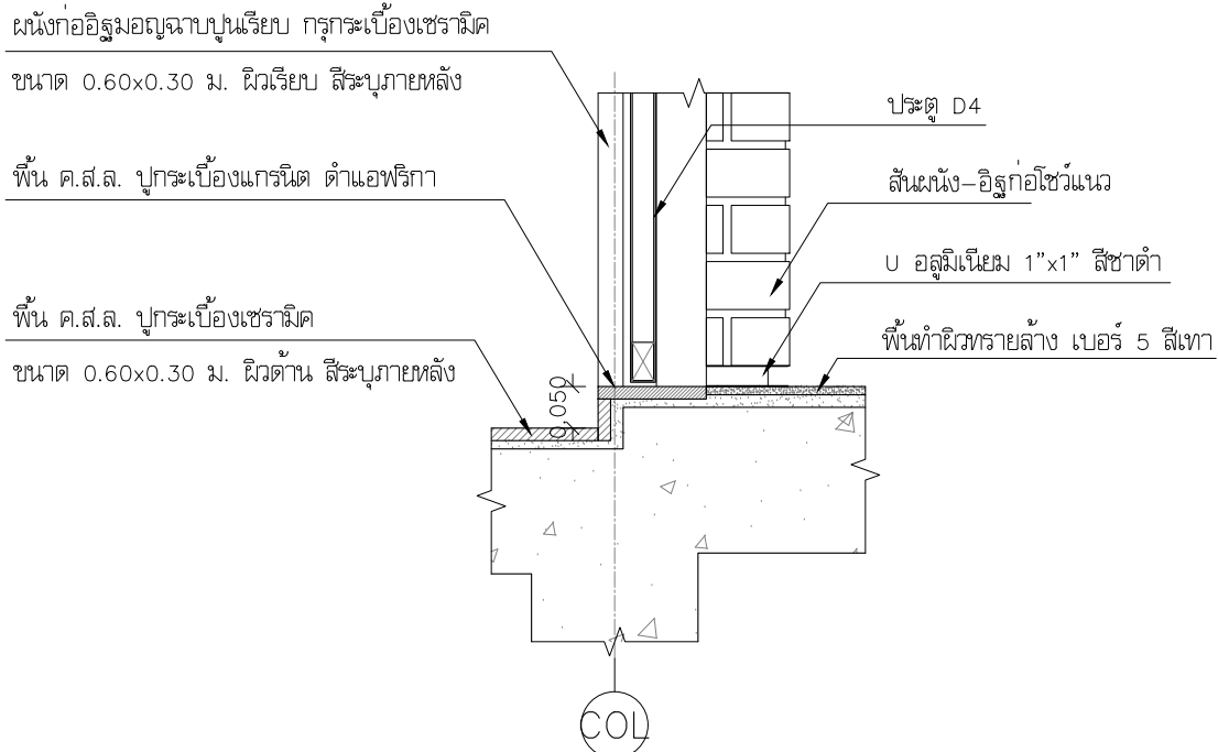
แบบขยาย ธรณีประตูห้องน้ำ มาตราส่วน 1:10
