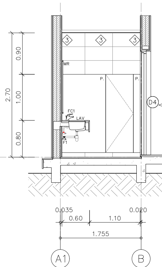
แบบขยายห้องน้ำ รูปตัด มาตราส่วน 1:50
