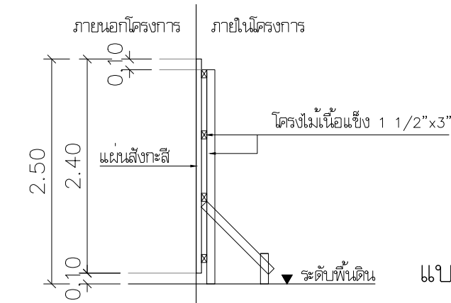
แบบขยายแนวผ้าใบกันวัสดุตกหล่น
