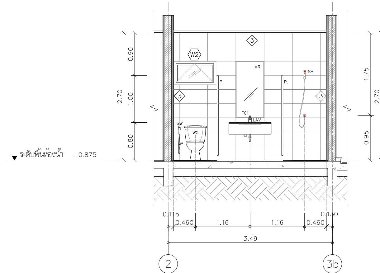
แบบขยายห้องน้ำ รูปตัด มาตราส่วน 1:50
