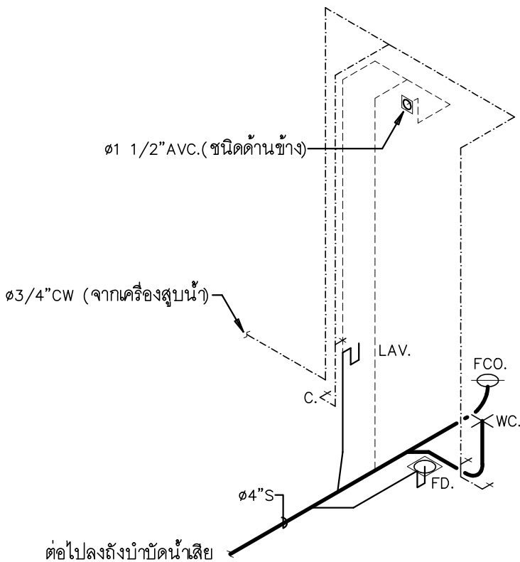
ไอโซเมตริกระบบสุขาภิบาลห้องน้ำ scale
