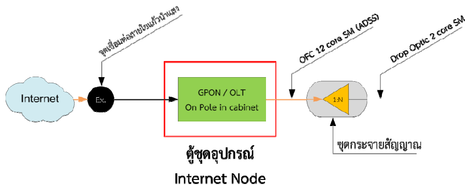
ภาพที่ 3 การติดตั้งและเชื่อมสัญญาณผ่านโครงข่ายภาคพื้นดิน ในจุดติดตั้งที่มีไฟฟ้า
