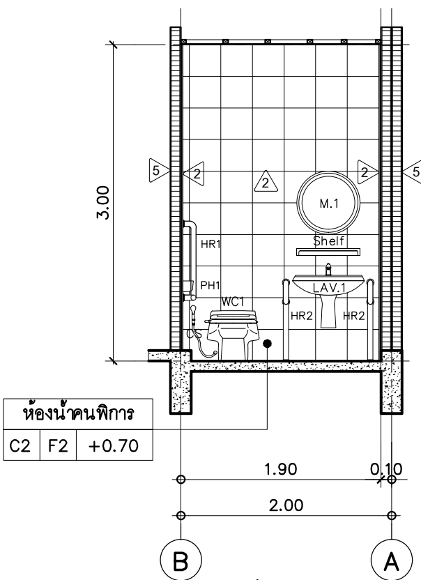
รูปตัด G scale 1: 50 (ห้องน้ำ- ส้วมคนพิการ)
