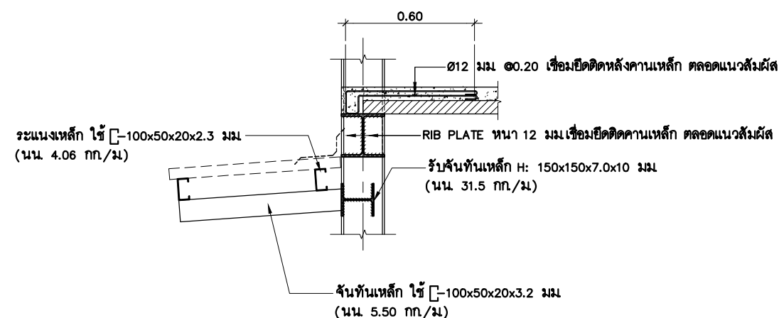
แบบขยาย TA 1:25
