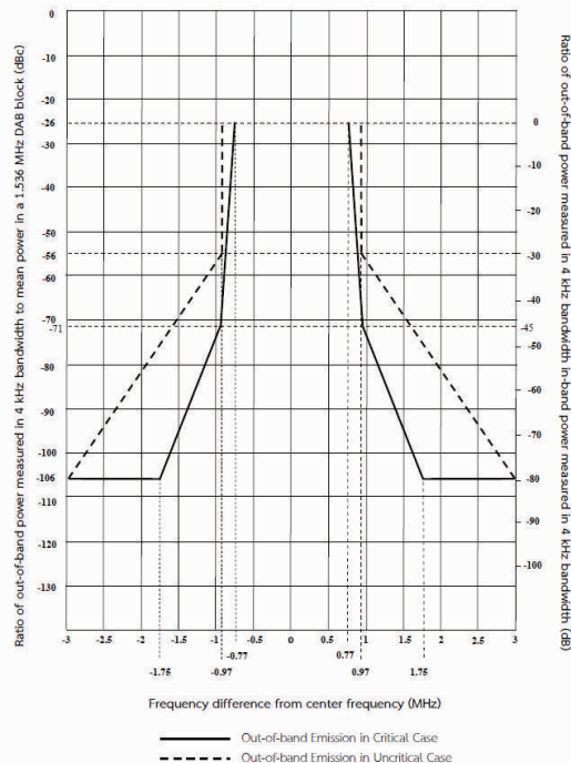
รูปที่ ๓ ขอบเขตการแพร่รบกวนแถบ
