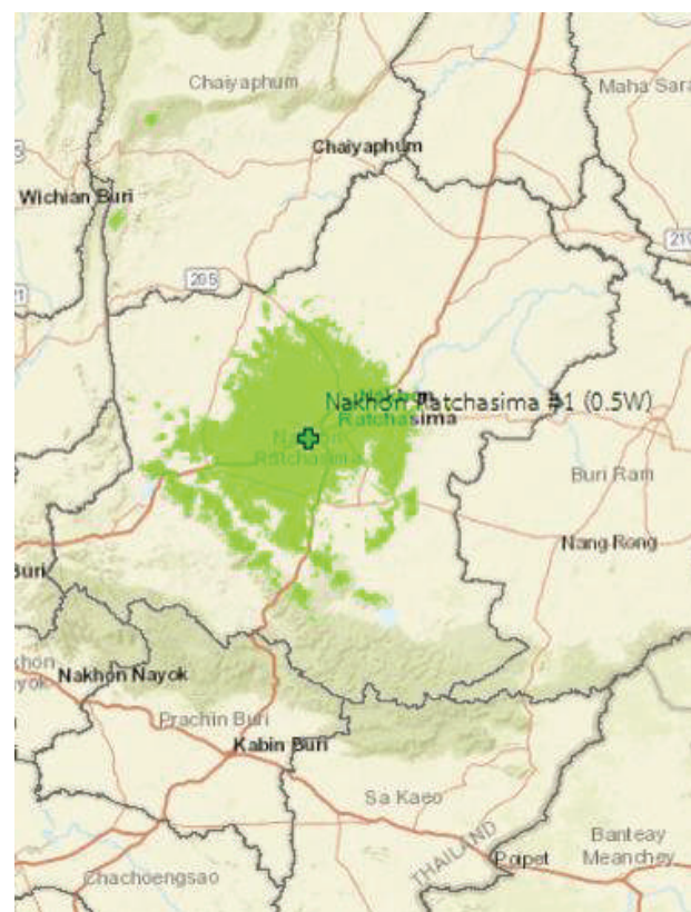
รูปที่ 9 พื้นที่การกระจายเสียงอ้างอิงของสถานีวิทยุคมนาคม Nakhon Ratchasima - N1
