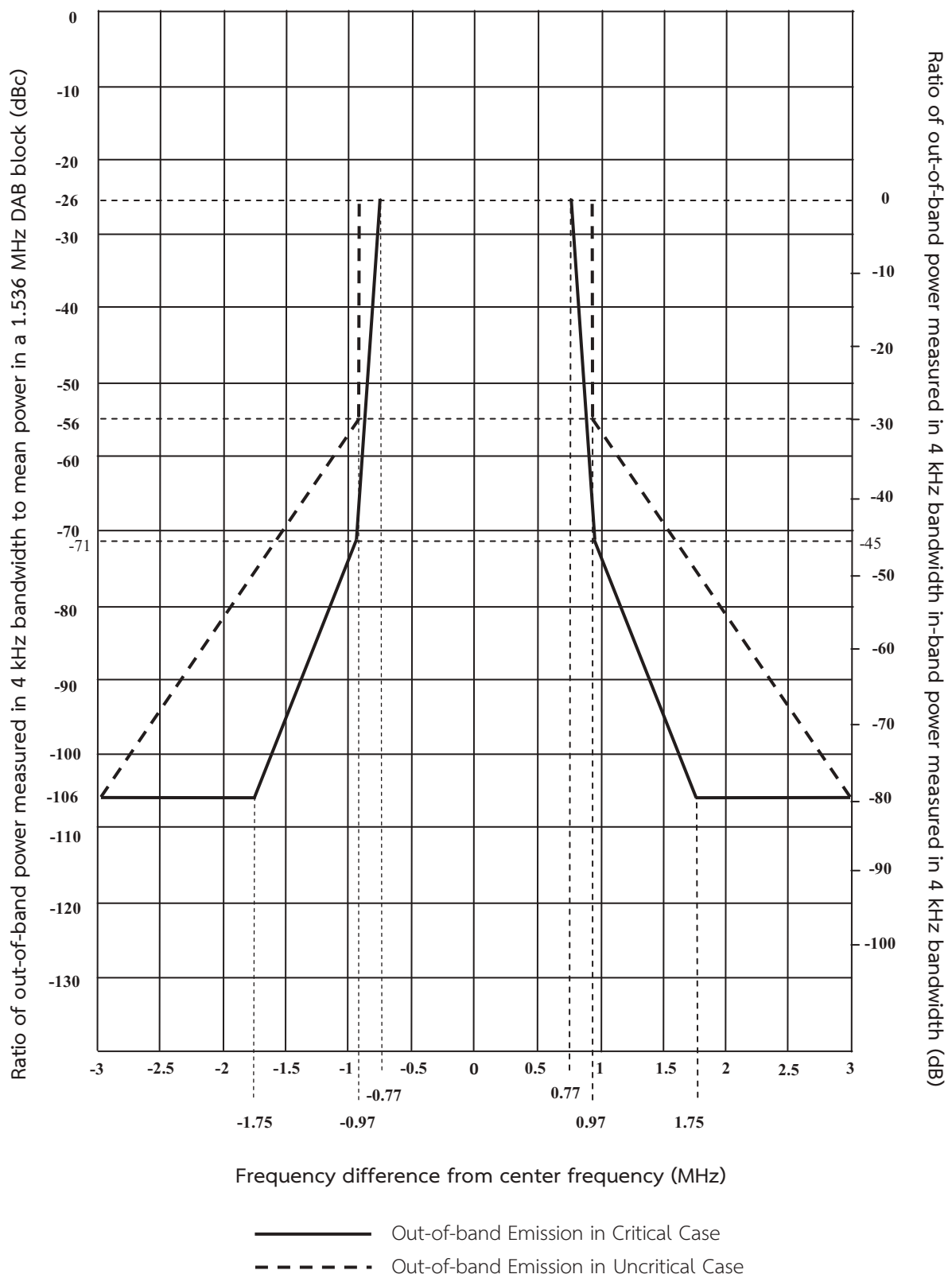
รูปที่ 3 ขอบเขตการแพร่รบกวน
