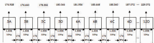
รูปที่ ๑ การกำหนดช่องความถี่วิทยุ
