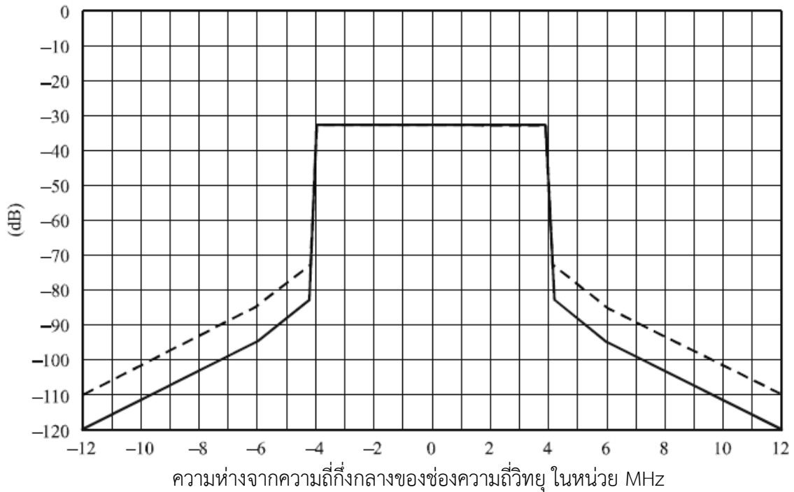
รูปที่ 1 กรอบของการแพร่กระจายคลื่น (Spectrum Mask)
