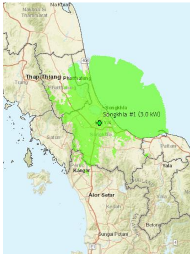
รูปที่ 13 พื้นที่การกระจายเสียงอ้างอิงของสถานีวิद्यุคมนาคม Song Khla - N1
