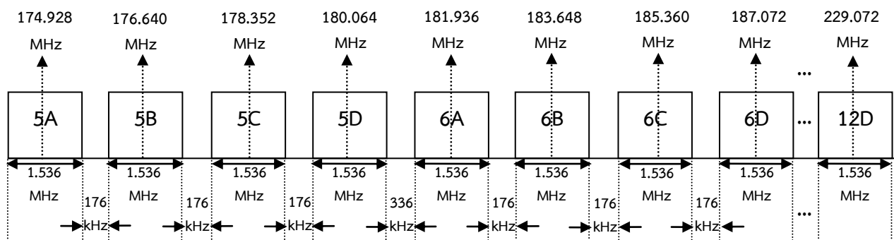
รูปที่ 1 แผนภาพบล็อกความถี่วิทยุ ความถี่วิทยุกึ่งกลาง ความกว้างแถบคลื่นความถี่ และความกว้างแถบคลื่นความถี่ป้องกัน
